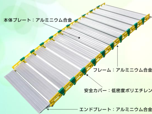
エンドプレート：アルミニウム合金
