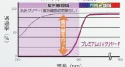
プレミアムUVクリヤーFは、汎用クリヤーと比較して紫外線を効率よくカットするため、紫外線劣化から基材の塗膜表面の劣化を抑制します。
